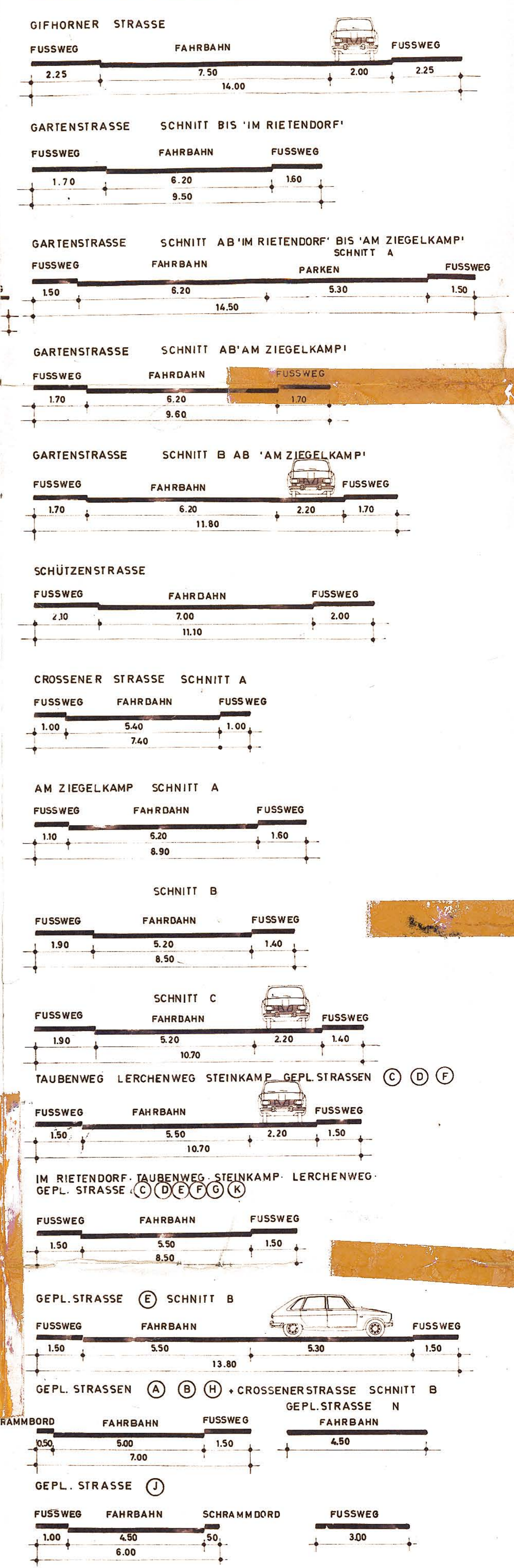
STRASSENQUERPROFILE M. 1:100
