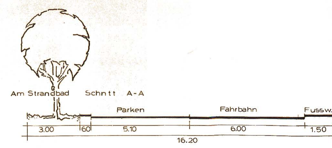
STRASSEQUERPROFILE M 1:100
